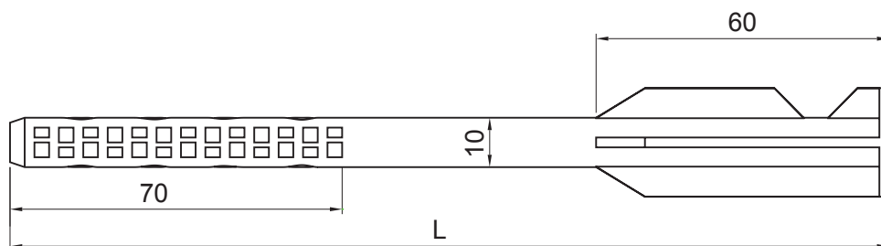
PREDNÝ POHĽAD
